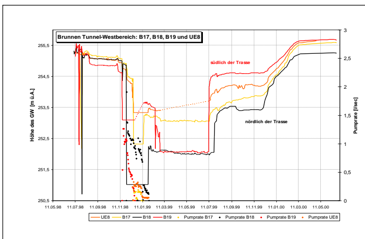
Grundwasserganglinien die die Wirksamkeit der Düker belegen.
